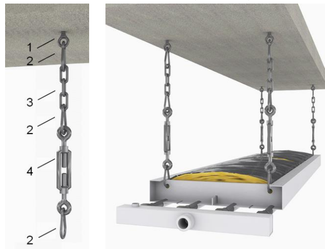
Крепление к бетонному потолку
