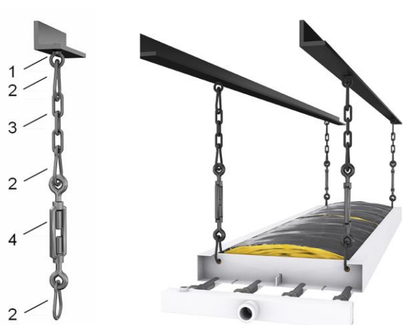
Крепление к уголку
